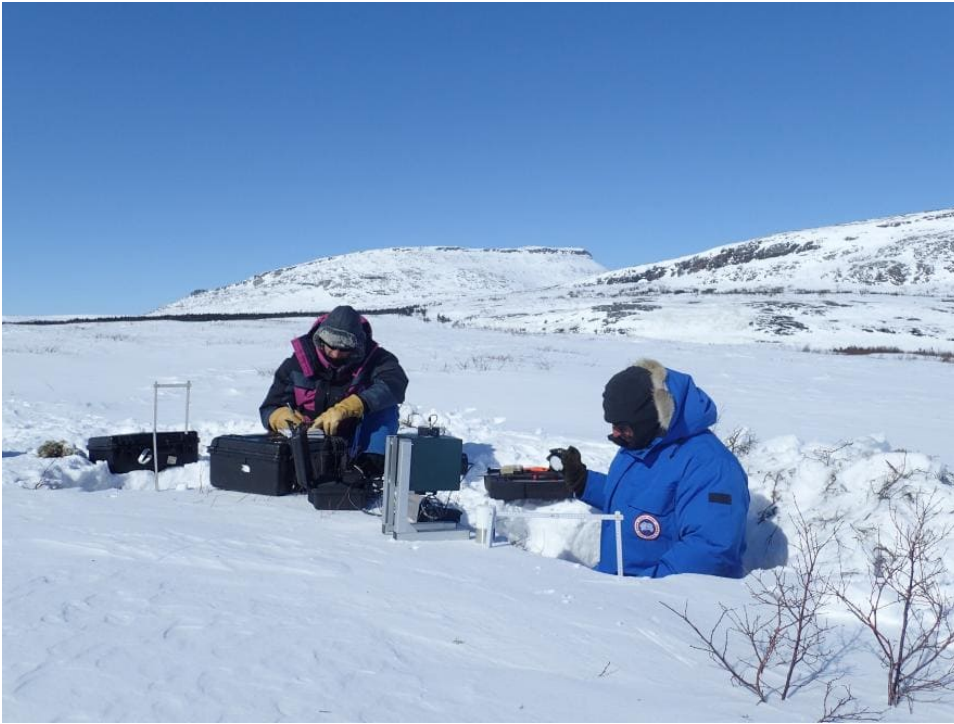
Florent Dominé (à droite) mesure les propriétés physiques de la neige avec son étudiant, Mathieu Barrère, près du village inuit d'Umiujaq, sur la côte Est de la baie d'Hudson (Canada). photographie de Florent Dominé
